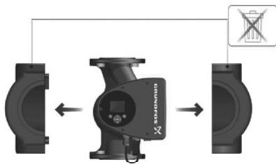
Рис. 4 Теплоизоляционные кожухи
