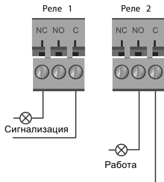
Рис. 23 Релейный выход
