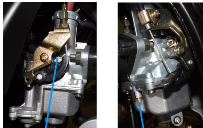
Винт количества
