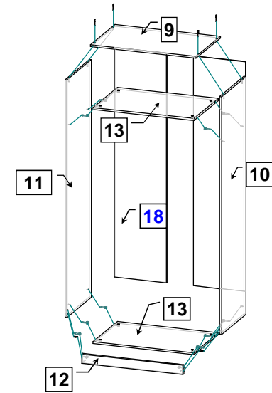
Шкаф для одежды 06.216 (собирается на правую и левую стороны)
