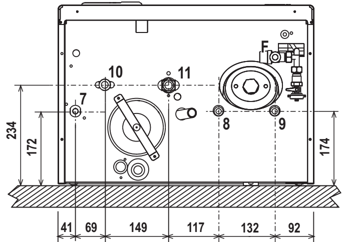
fig. 13 - Conexiones hidráulicas
