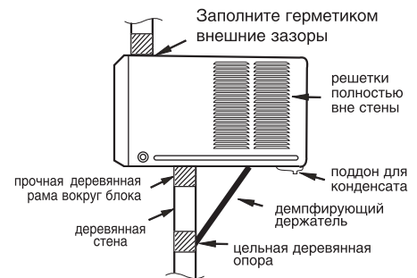
способ монтажа кондиционера для случая, когда нельзя сделать внешнюю опору
