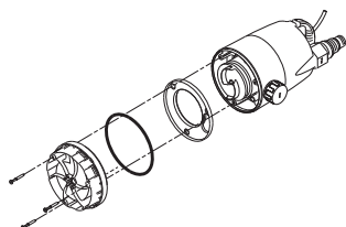
Рис. 12 Демонтаж деталей, находящихся в днище насоса
