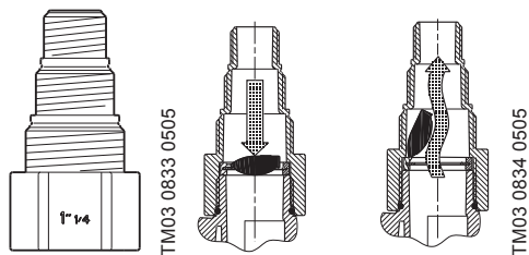
Рис. 6 Переходник и обратный клапан (положение и функция)
