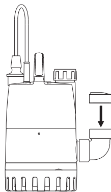
Рис. 7 Правильное положение обратного клапана
