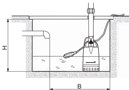
Рис. 3 Минимальные монтажные размеры
