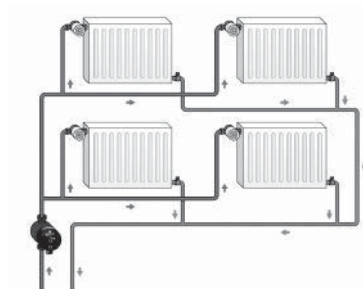
Рис. 5 Двухтрубная система отопления
