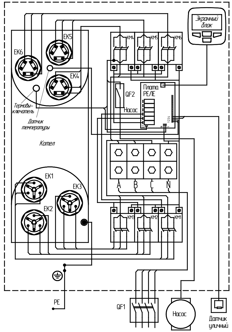
Рисунок 9. Схема подключения ЭВАН UNIVERSAL -66 - 15 -
