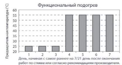
Рис. 15. Функциональный подогрев
