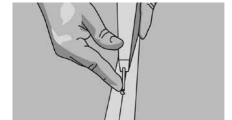
Рис. 43. Всегда работайте двумя руками! Одной рукой держите тубик, указательный палец второй руки положите на сопло. Вдавите иглу глубоко в шов так, чтобы холодная сварка попала в образовавшееся отверстие.
