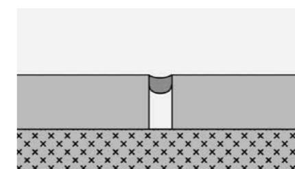
Рис. 33. Площадь контакта сварочного шнура и покрытия слишком маленькая. При этом прочность сваренного шнура примерно 10-15 N/CM.
