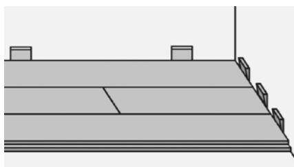
Рис. 106. Перед приклеиванием проведите подрезку и пробную сборку трех первых рядов без клея. С каждой стороны ряда необходимо оставить компенсационный зазор (10-15 мм.), в который устанавливаются расширительные клинья.
