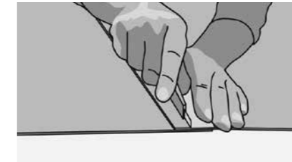
Рис. 38. Положить полотнища внахлест (3-5 см) и разрезать одновременно два полотнища по металлической планке.
