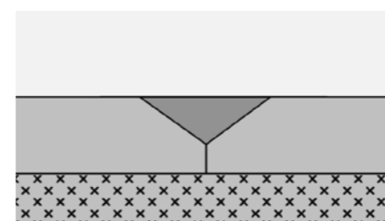
Рис. 31. Большая площадь контакта сварочного шнура и покрытия. При этом прочность сваренного шнура примерно 140 N/CM.
