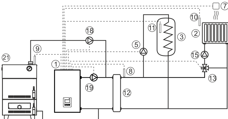
Рис.7 Упрощенная схема подключения котла в режиме вспомогательного с гидрозделителем.
