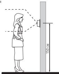
Рис. 4 Рекомендуемая высота установки видеопанели
