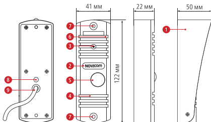
Рис. 2 Вызывная панель LEGEND
