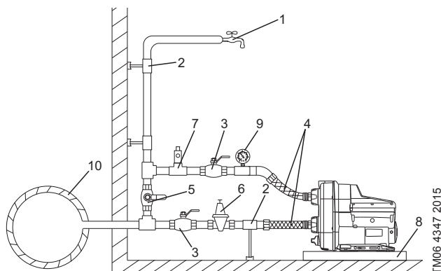
Рис. 8 Повышение давления воды из магистрального трубопровода
