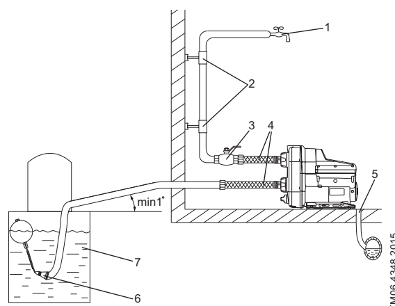
Рис. 10 Подача воды из резервуара
