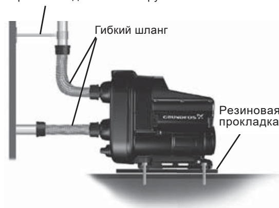
Рис. 7 Мероприятия по уменьшению шума для SCALA2
