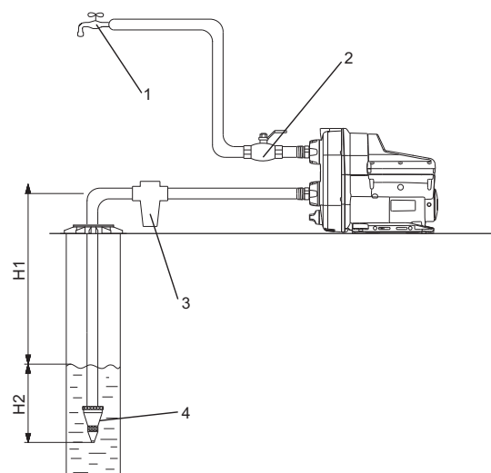
Рис. 9 Подача воды из колодца/скважины
