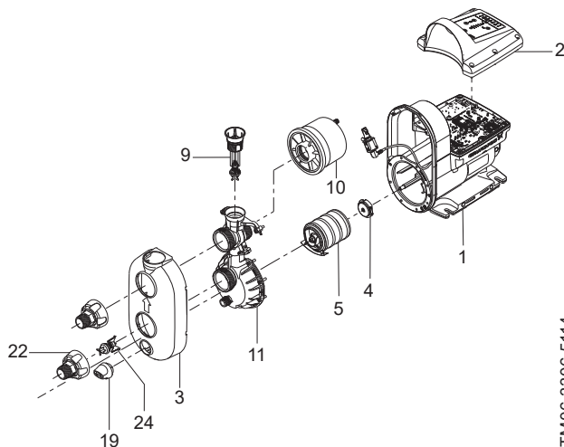
Рис. 2 Конструкция SCALA2
