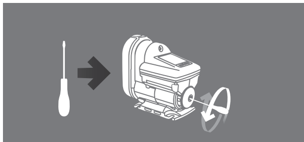
Рис. 17 Разблокировка вала насосной установки SCALA2
