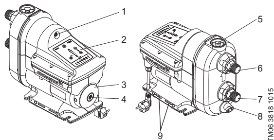
Рис. 1 Внешний вид SCALA2
