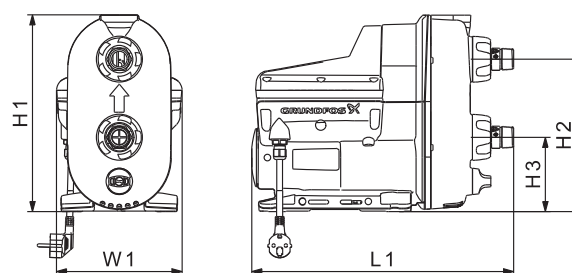
Рис. 22 Габаритный чертёж SCALA2
