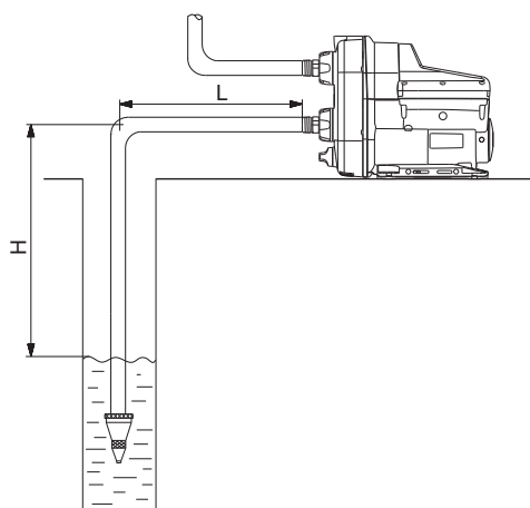
Рис. 11 Длина всасывающего трубопровода
