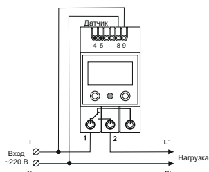
Схема подключения
