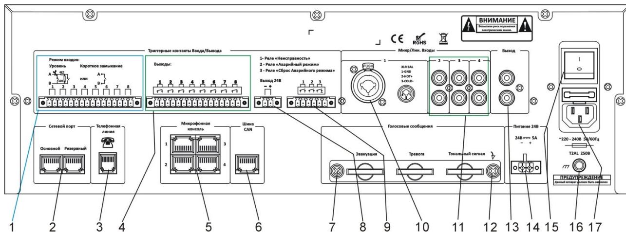
Рис. 3.3. Задняя панель контроллера LPA-EVA-MA
