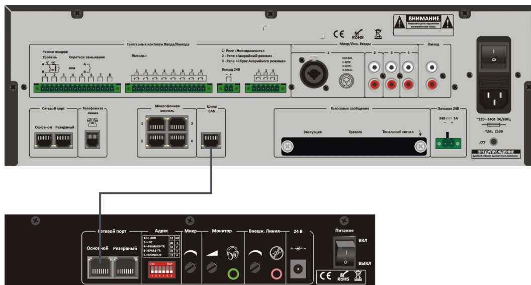
Рис. 4.46. Неправильное соединение микрофонной консоли LPA-EVA-RM и контроллера LPA-EVA-MA
