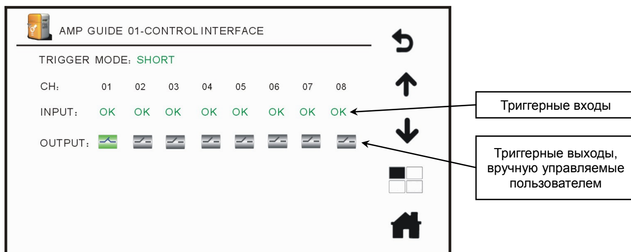
Рис. 4.14. Интерфейс управляющих сигналов коммутатора усилителей
