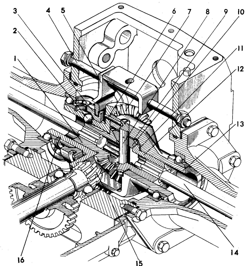
Рисунок 11 – Ведущий мост
