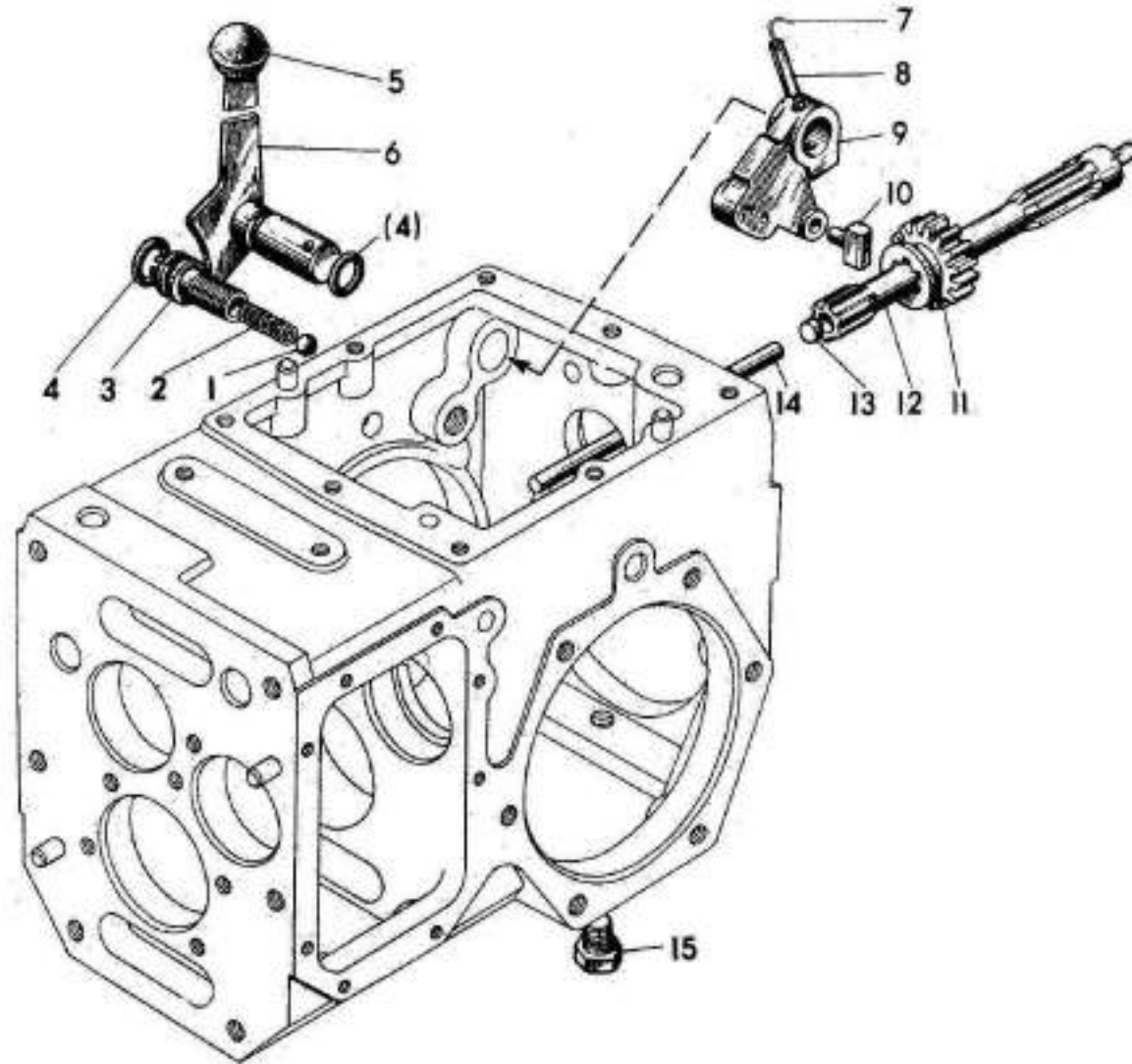
Рисунок 11 – Управление и привод ВОМ
