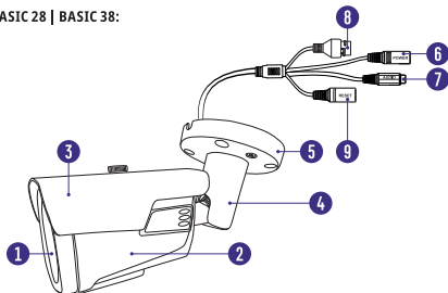
Рис. 6 Описание камеры BASIC 28 | BASIC 38
