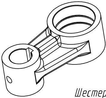
Серьга С52.20.00.03
