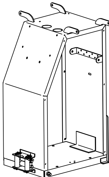
Корпус ТН190.08.000
