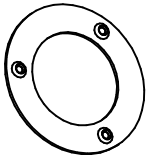
Кольцо ТН190.03.003
