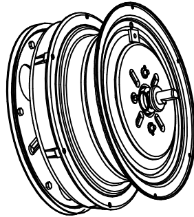
Барaban ТН190.03.000
