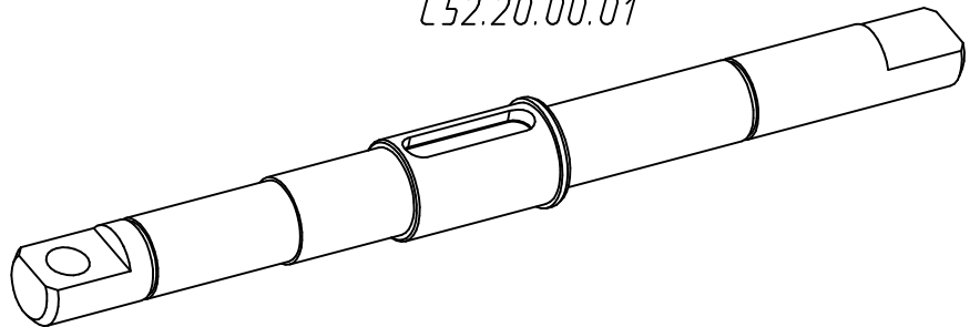
Вал С52.20.00.01
