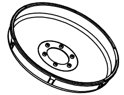
Крышка ТН190.03.002 (Граднамид марки ПА6-ЛТ-СВ30, ТУ РБ 500048054.020-2001 )
