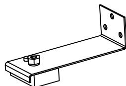
Колодка С52.140.00.00
