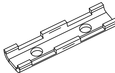
Прижим С52.00.00.34
