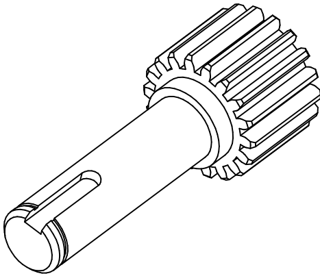
Палец С52.20.00.12
