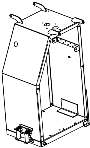
Корпус С52.10.00.00
