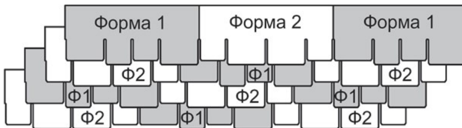
Рис. 5 Схема чередования гонтов гибкой битумной черепицы Döcke PIE коллекции Саппоро.
