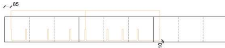
Рис. 4. Укладка первого ряда рядовой черепицы коллекции САППОРО.
