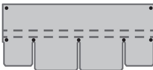
Рис. 2б. Гибкая битумная черепица коллекции САППОРО ФОРМА 2.
