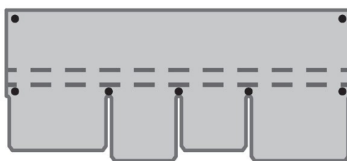
Рис. 2а. Гибкая битумная черепица коллекции САППОРО ФОРМА 1.
