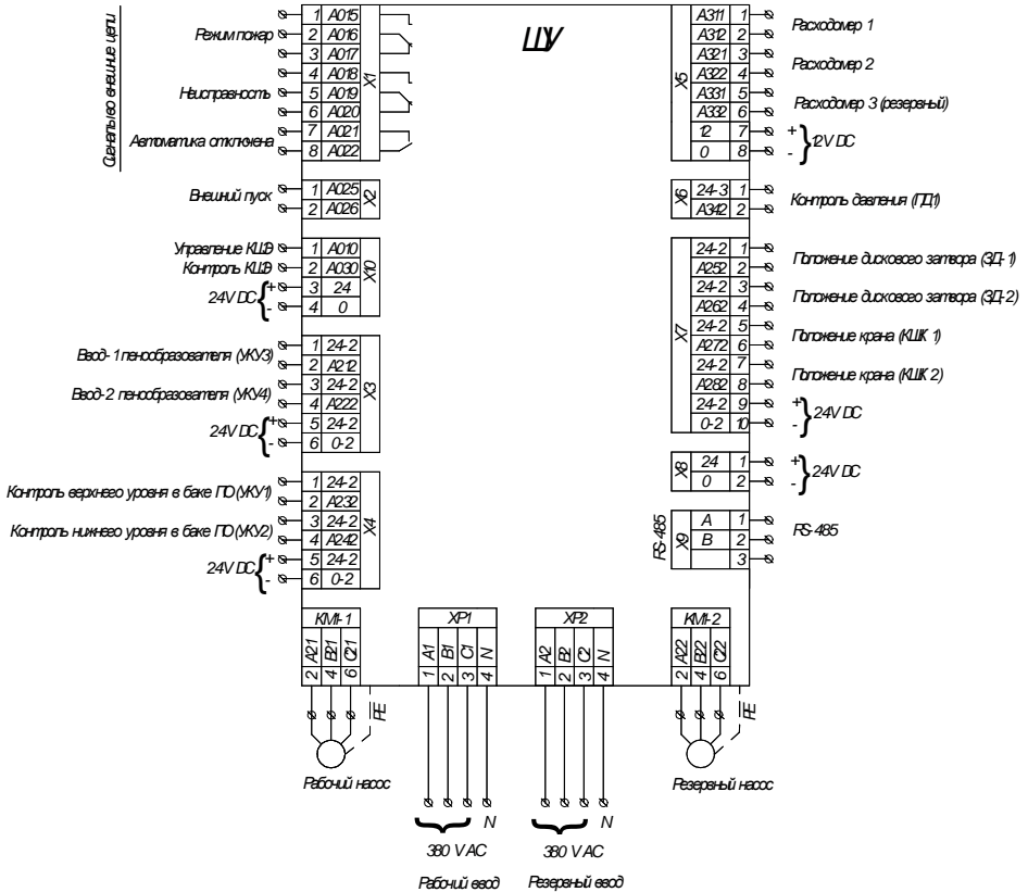
Рисунок Б.2 – Схема внешних подключений ШУ
