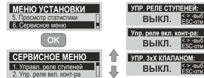
Рисунок 33. Сервисное меню.
