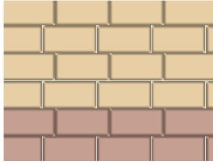
Трехчетвертная перевязка
