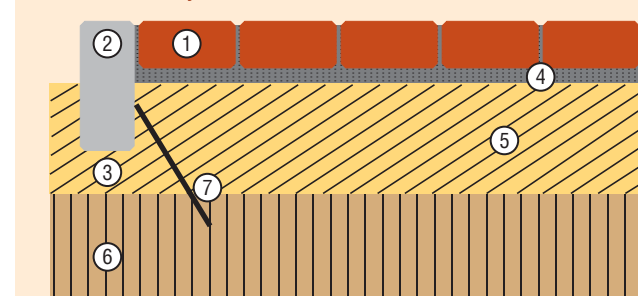
Рисунок №3. Водоотвод из монтажного слоя.
