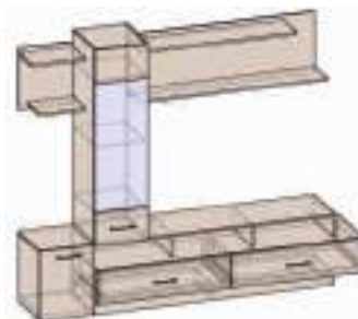
Аризона-8 Ш2060 В1694 Г440 max TV размер В1200 Ш808
