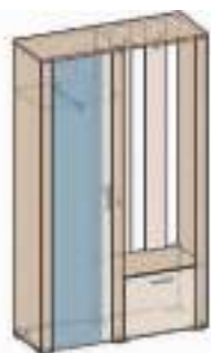
Шкаф с зеркалом и вешалкой (левый) КЛ-14Л ШД170 В2020 Г425
