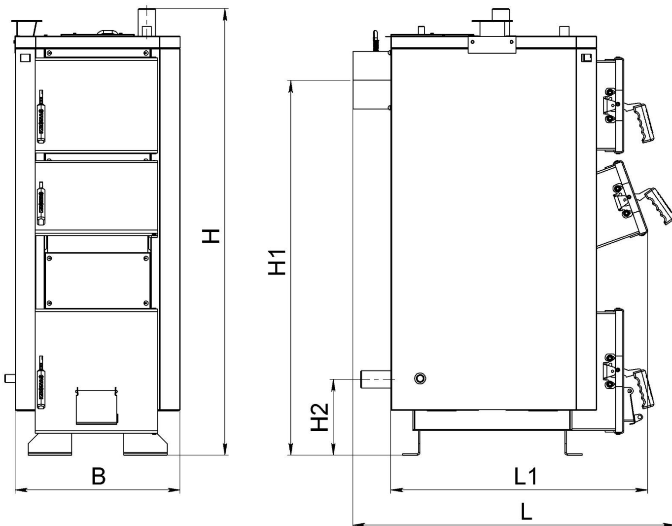
Рисунок 3.1 – Позначення габаритів котла типу КТК (потужністю 15-30 кВт)
