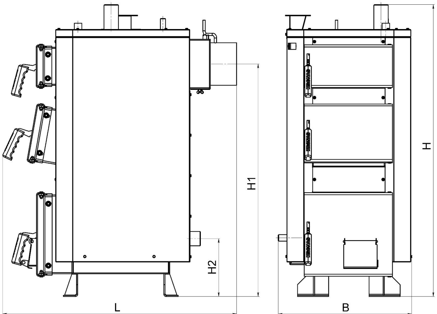
Рисунок 3.1 – Позначення габаритів
