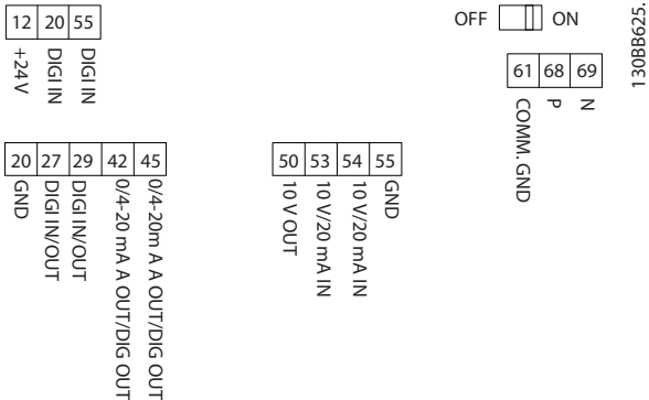
Рисунок 4.11 Клеммы управления
