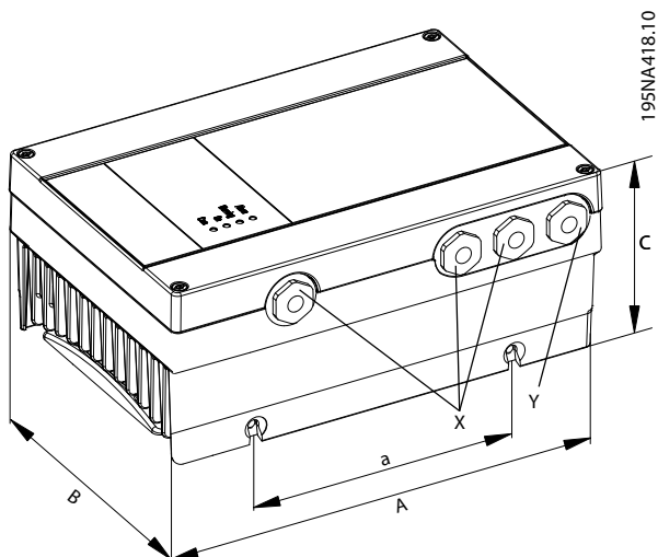
Рисунок 7.2 Размеры FCP 106
