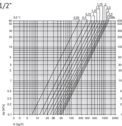
Гидравлическая характеристика D1/2"
