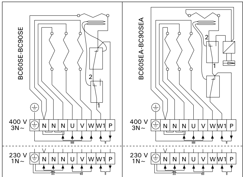
Рисунок 8. Электромонтаж каменки
