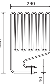
ZSP-250 2500W/230V F15, F16,5, K13,5G/S, K15G/S PO165
