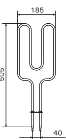
ZSA-420 250W/230V AV2, AV4, AV6
