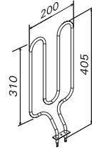
ZSN-150 1150W/230V D23/E, D23EE, D29EE
