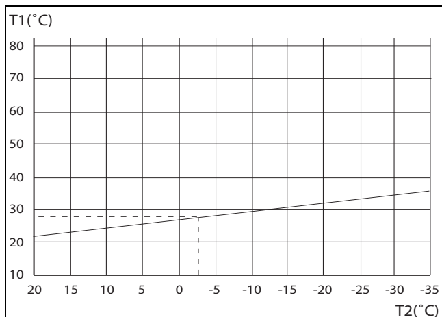
Рис. 22 Обогрев пола
