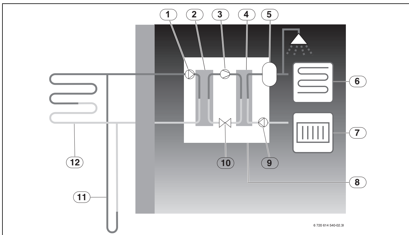
Рис. 2 Принцип действия
