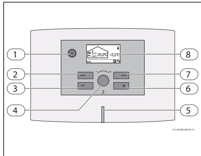
Рис. 3 Панель управления
