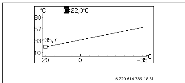
Рис. 23 Настройка отопительной кривой (отопления)
