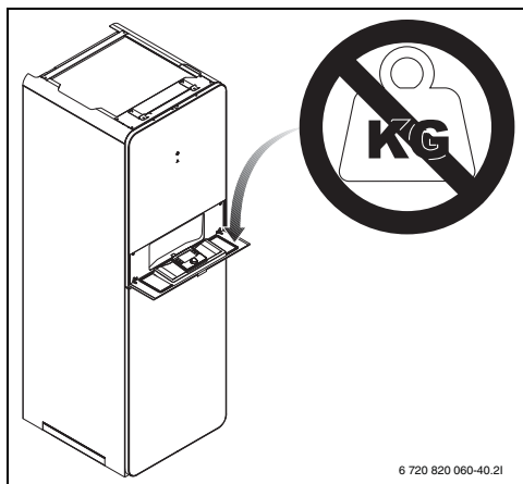
Рис. 9 Пульт управления AWM/AWMS
