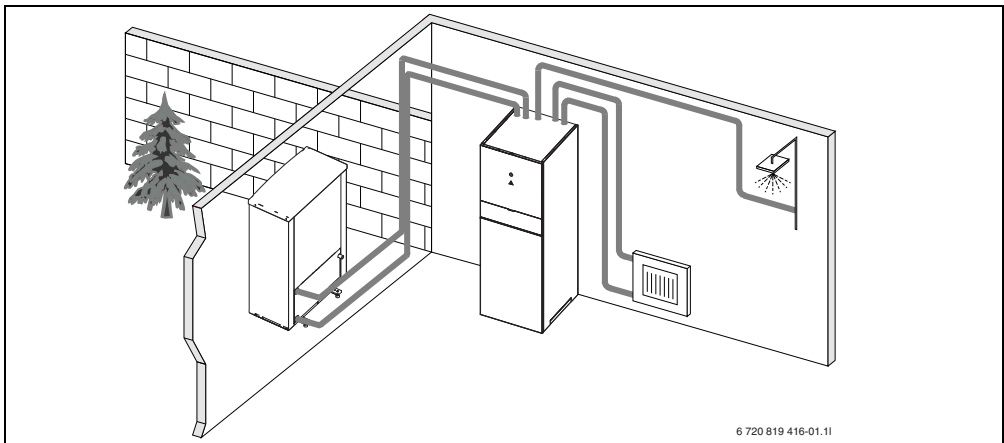
Рис. 1 Тепловой насос CS7000i AW, компактный блок AWM/AWMS со встроенным баком-водонагревателем и электрическим нагревателем
