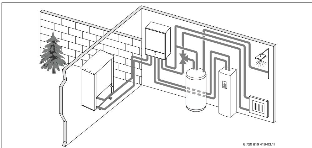
Рис. 3 Тепловой насос CS7000i AW, компактный блок AWB без электрического нагревателя, отдельный бак-водонагреватель и отдельный дополнительный нагреватель
