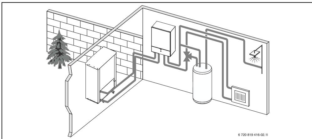
Рис. 2 Тепловой насос CS7000i AW, компактный блок AWM с электрическим нагревателем и отдельный бак-водонагреватель
