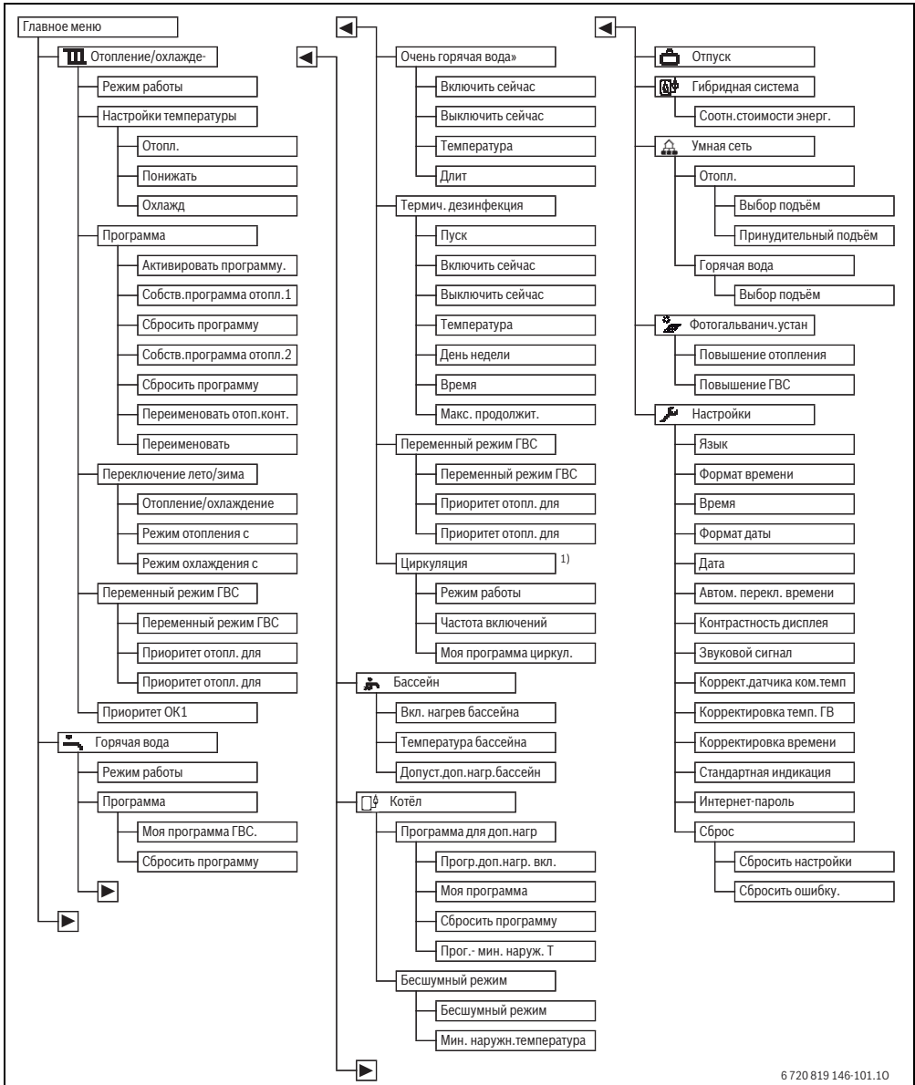
Рис. 12 Структура главного меню
