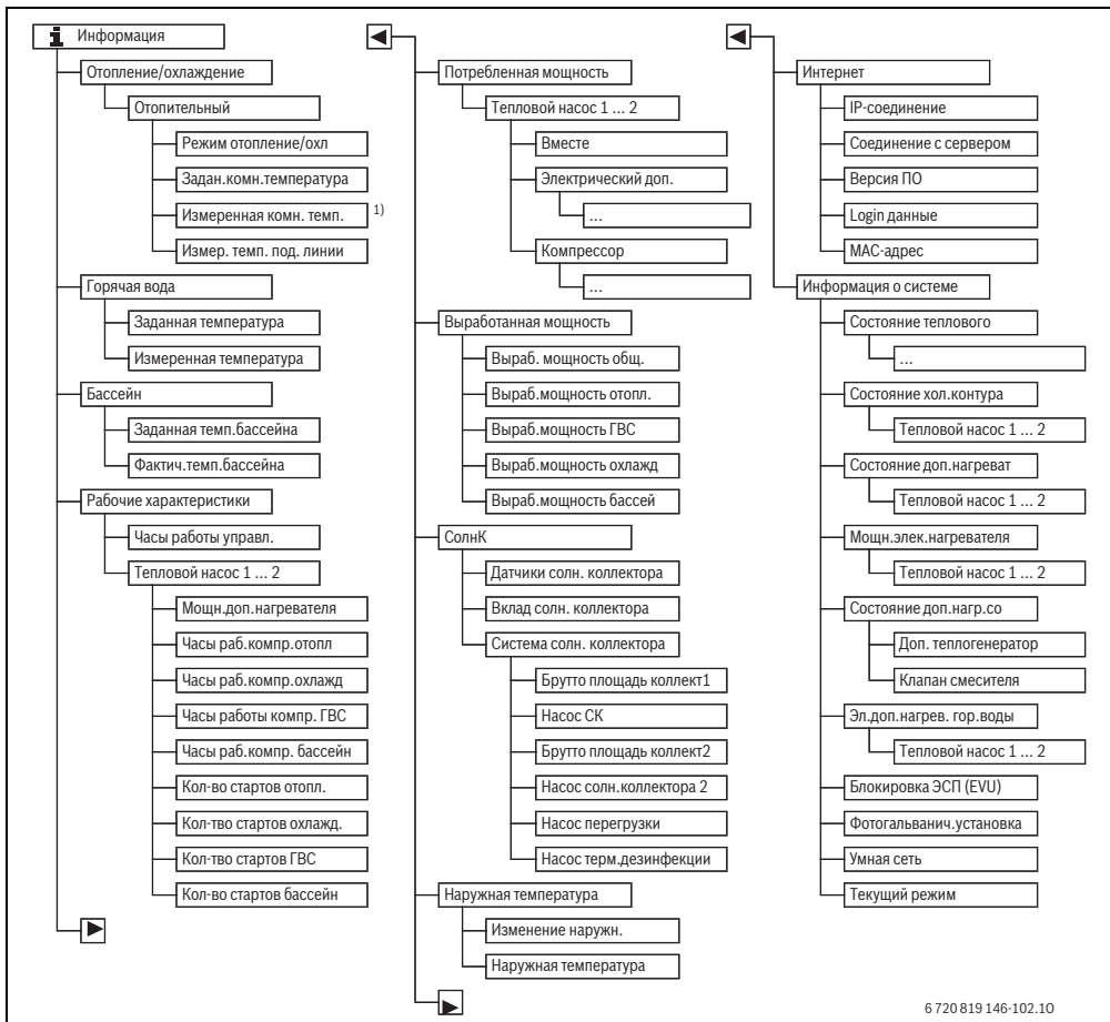
Рис. 14 Структура информационного меню
