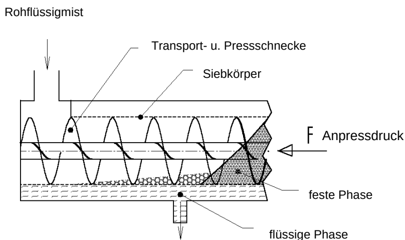
Abb. 3-1 Funktionsbeschreibung
