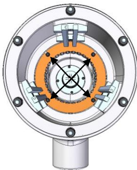
Abb. 13-8 Verschleißring
