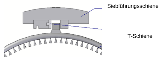
Abb. 13-6 T-Schiene
