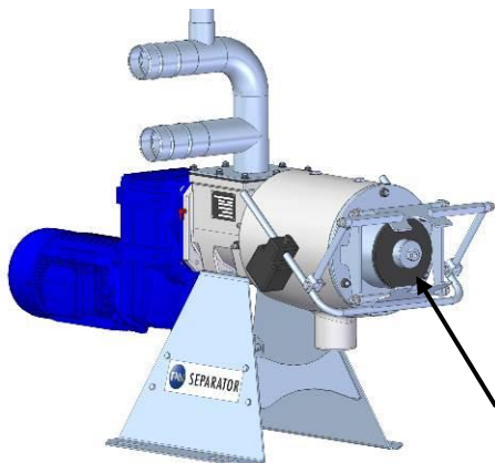
Abb. 7-3 Stopfenbildungshilfe
