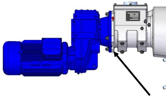
Abb.13-3 Kontrollöffnung
