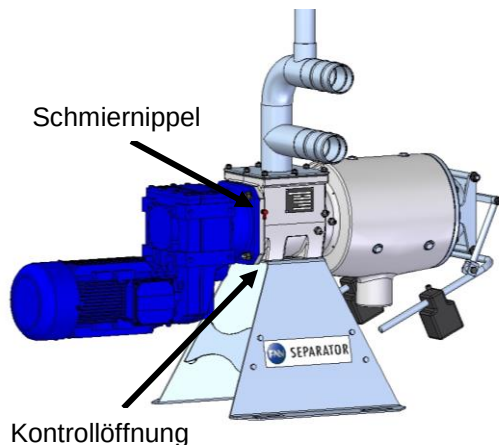
Abb. 13-1 Versorgung mit Sperrmedium
