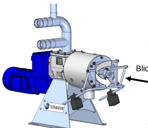
Abb. 5-1 Drehrichtung Schnecke
