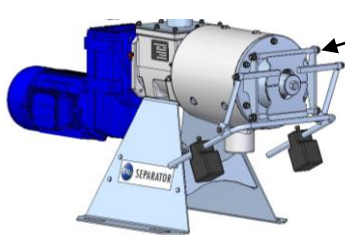
Abb. 7-2 Ausbringklappen
