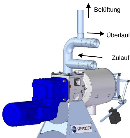
Abb.4-7 Einlauf-Aufbau
