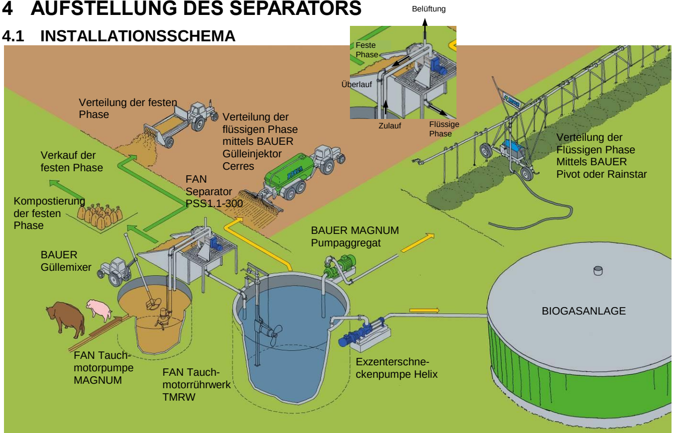
Abb. 4-1 Installationsschema
