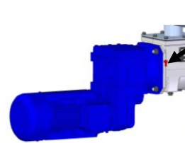
Abb. 13-2 Schmiernippel
