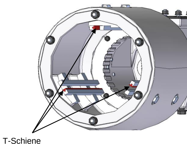
Abb. 13-5 Gehäuse Separator PSS 1.1-300 mit Siebführungsschienen und T-Kunststoffprofilschienen
