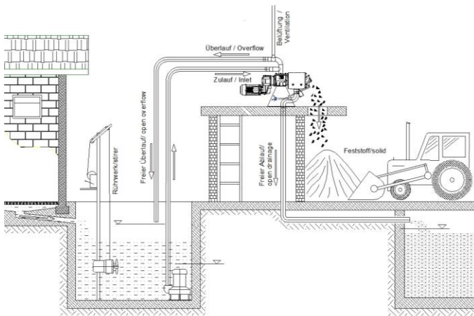
Abb.4-5 Beschickung über Pumpe
