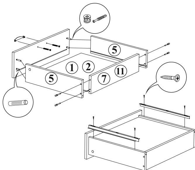
Сборка ящика
