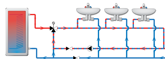
Схема 2. Клапан АТМ используется для поддержания постоянной (настроенной) температуры в контуре циркуляции горячей воды.
