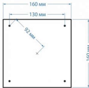
Основание светильника
