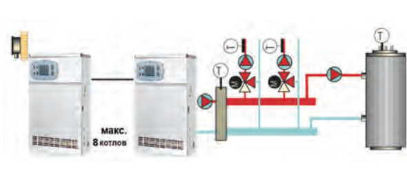
Каскадная установка
