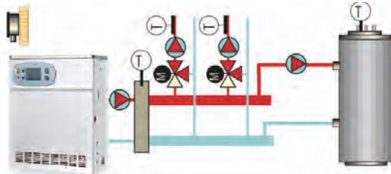
Единая установка
