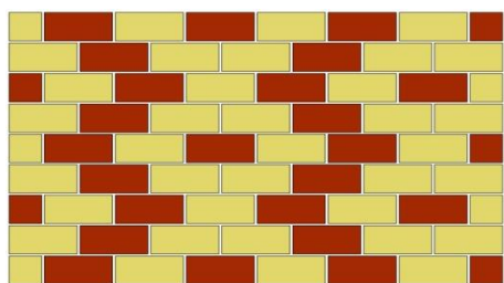
Половинная перевязка
