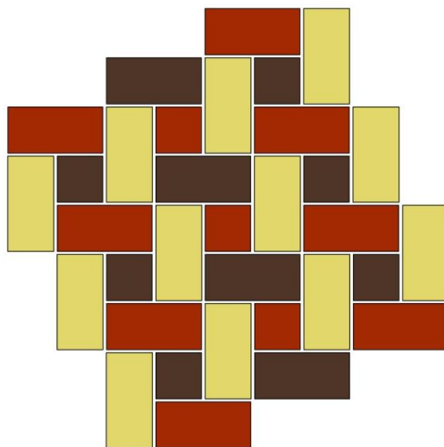
Винтовая перевязка с малой розеткой
