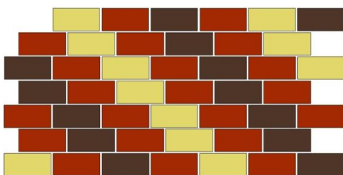
Трехчетверговая перевязка
