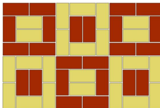
Винтовые большие перевязки
