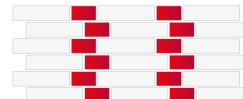
WIĄZANIE GOTYCKIE
