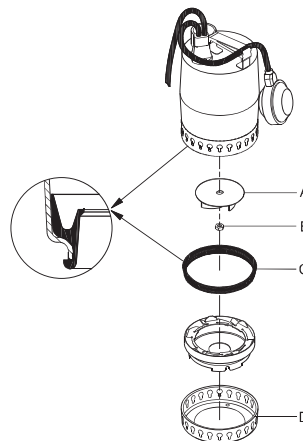
Рис. 15 Детали для технического обслуживания
