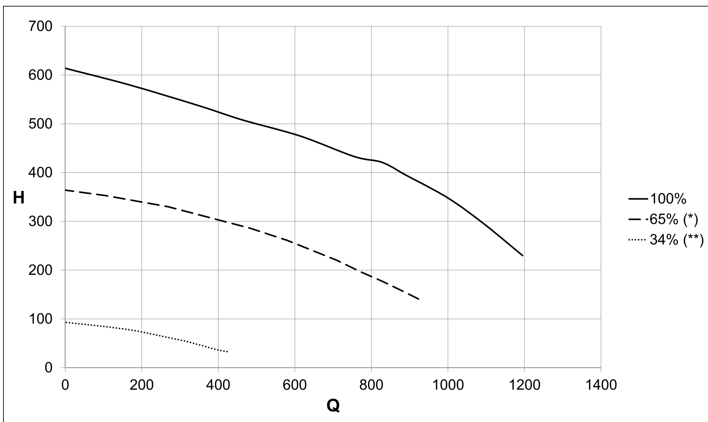
Рис. 22 Располагаемый напор KC-KR-KRB 28
