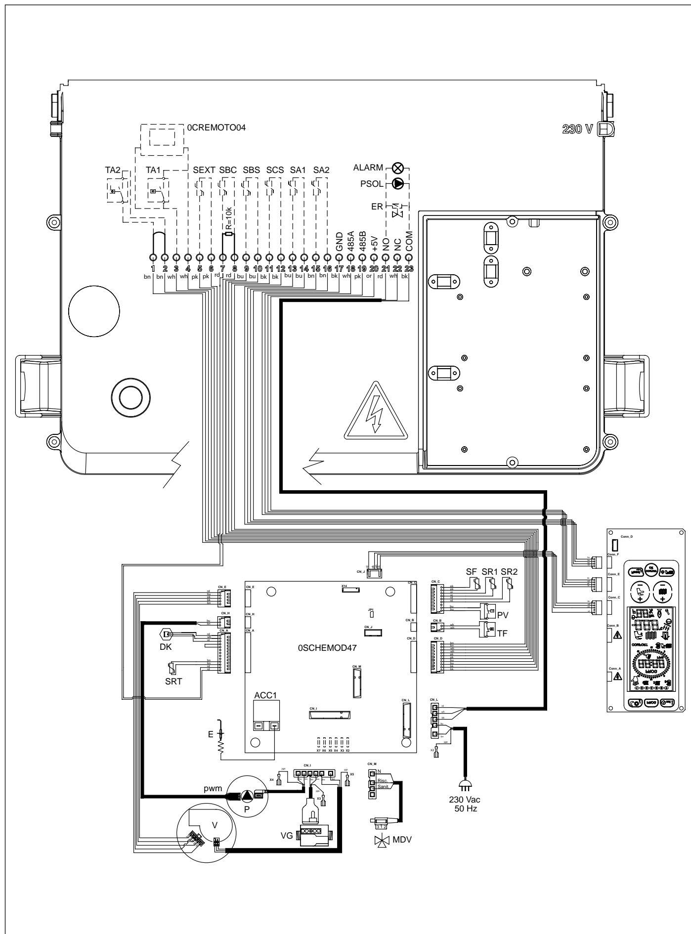
Рис. 32 Электрическая схема KRB
