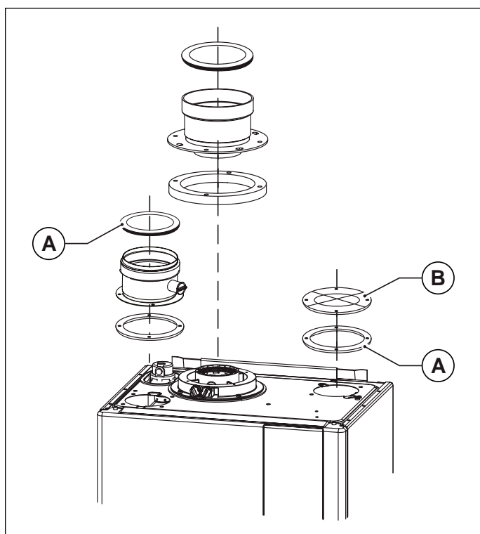
Рис. 13 Коаксиальная система воздухозабора и дымоотвода типа C43 - C53 - C83
