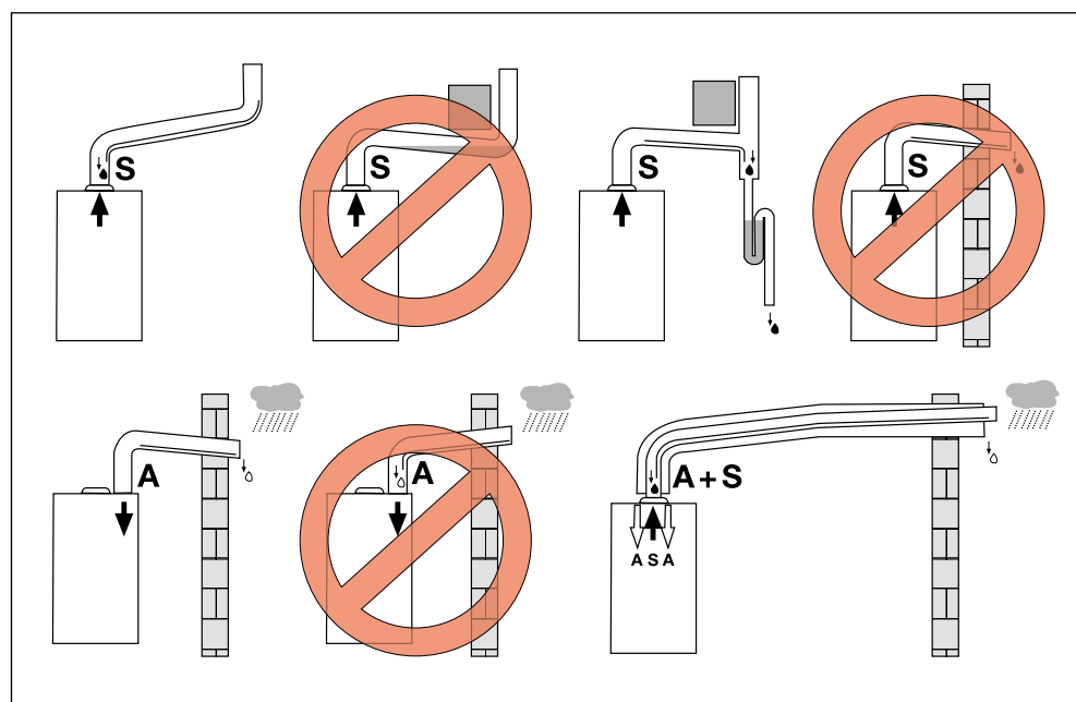
Рис. 10 Примеры установки
