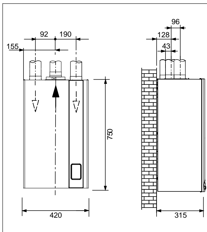
Рис. 14 Размеры для коаксиальных трубопроводов типа C43 - C53 - C83
