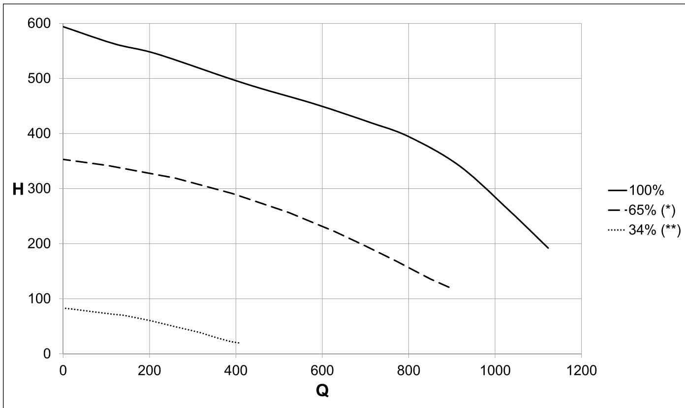
Рис. 21 Располагаемый напор KC-KR-KRB 24
