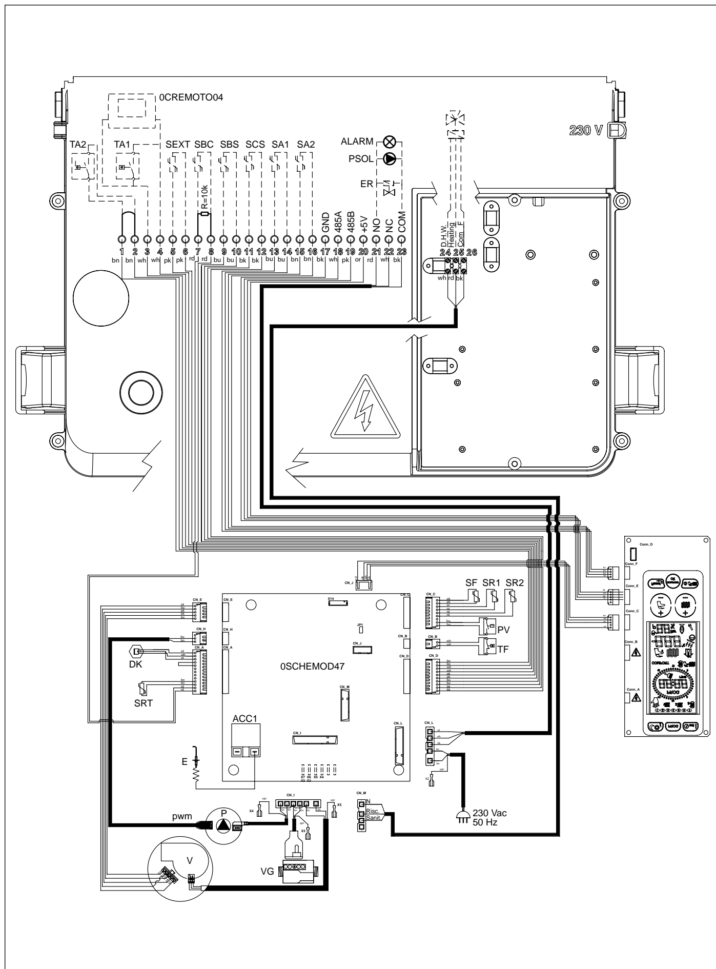
Рис. 29 Электрическая схема KR
