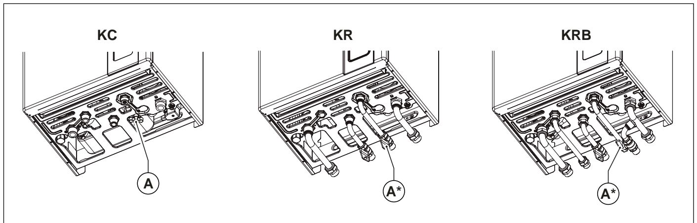
Рис. 2 Краны заполнения
