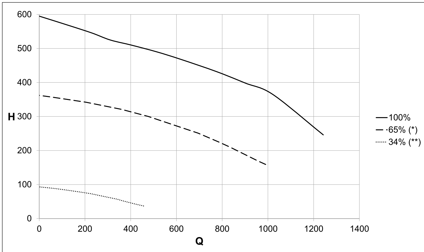
Рис. 23 Располагаемый напор KC-KR-KRB 32
