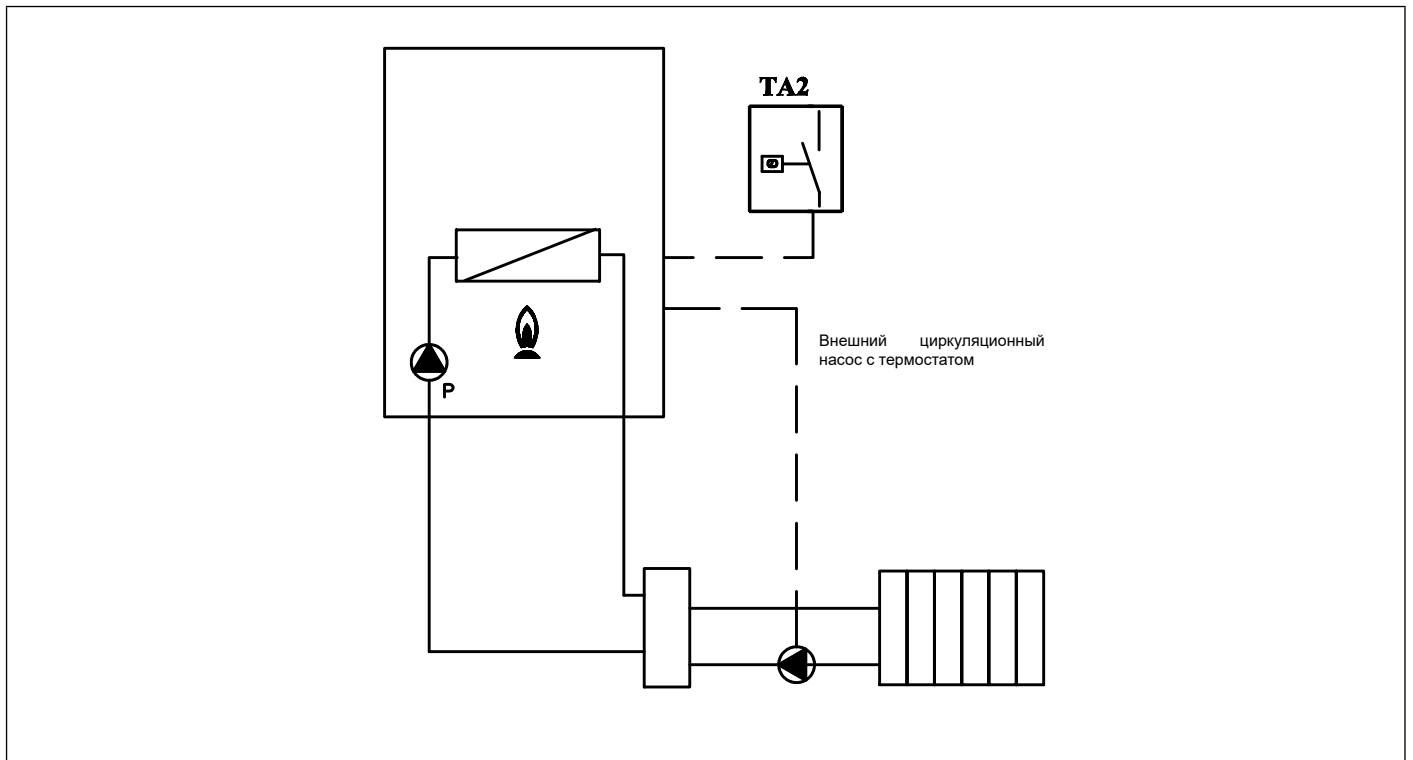
Рис. 35 Работа реле по внешнему запросу (P17=3)
