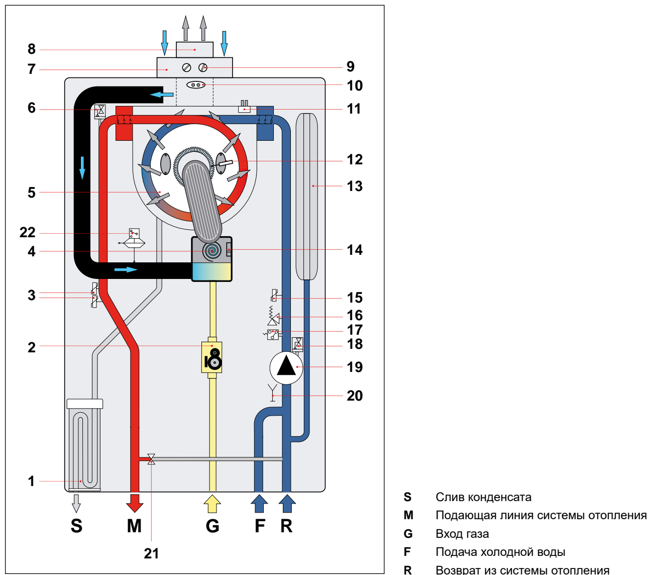
Рис. 7 Гидравлическая схемм мод. KR
