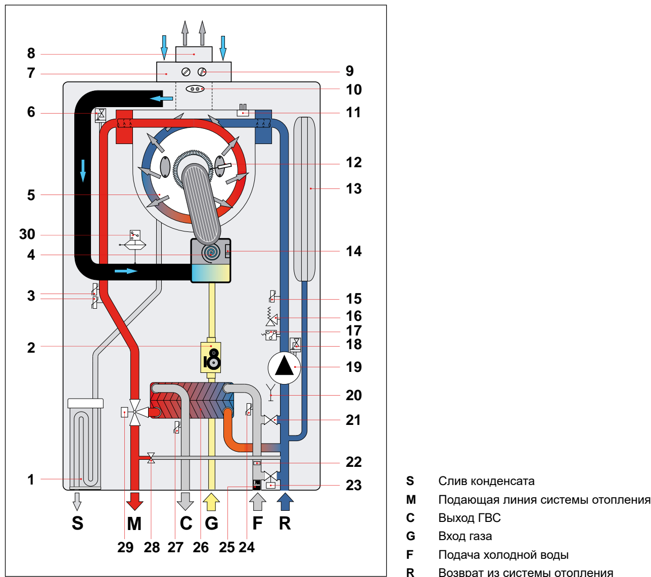
Рис. 6 Гидравлическая схемм мод. КС
