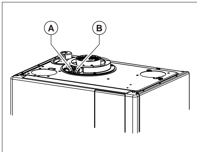
Рис. 15 Положение заглушек
