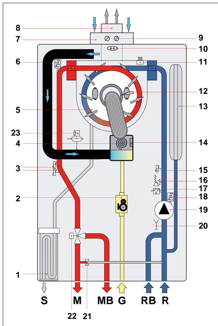
Рис. 8 Гидравлическая схемм мод. KRB
