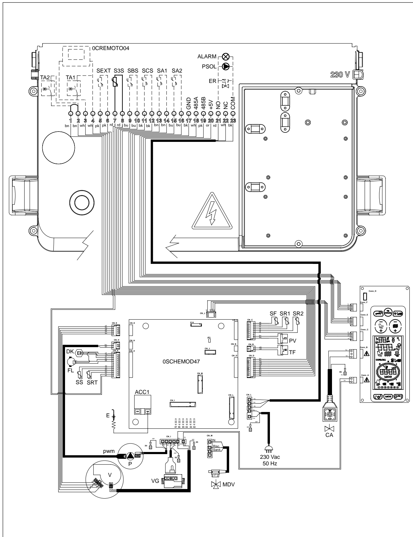
Рис. 24 Электрическая схема КС
