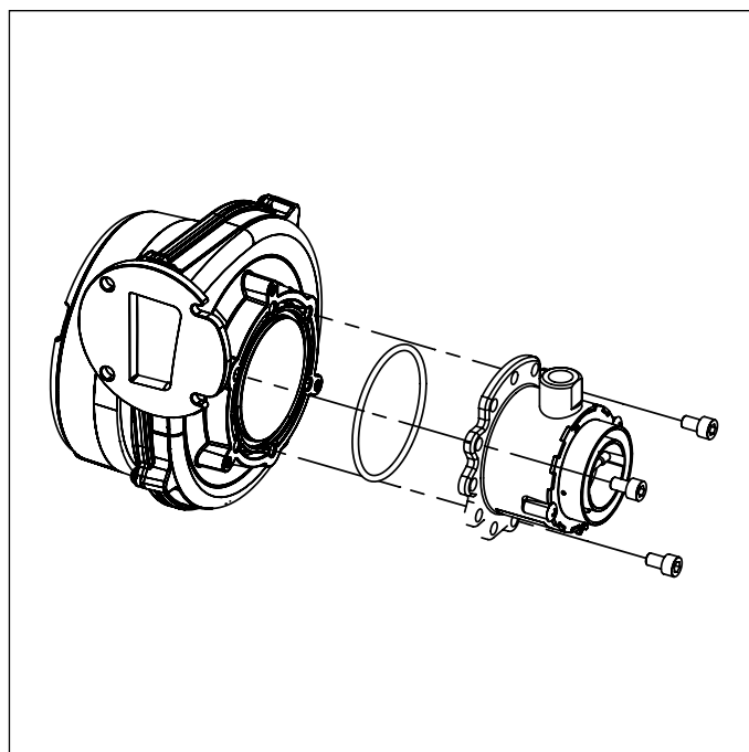
Рис. 37 Смеситель
