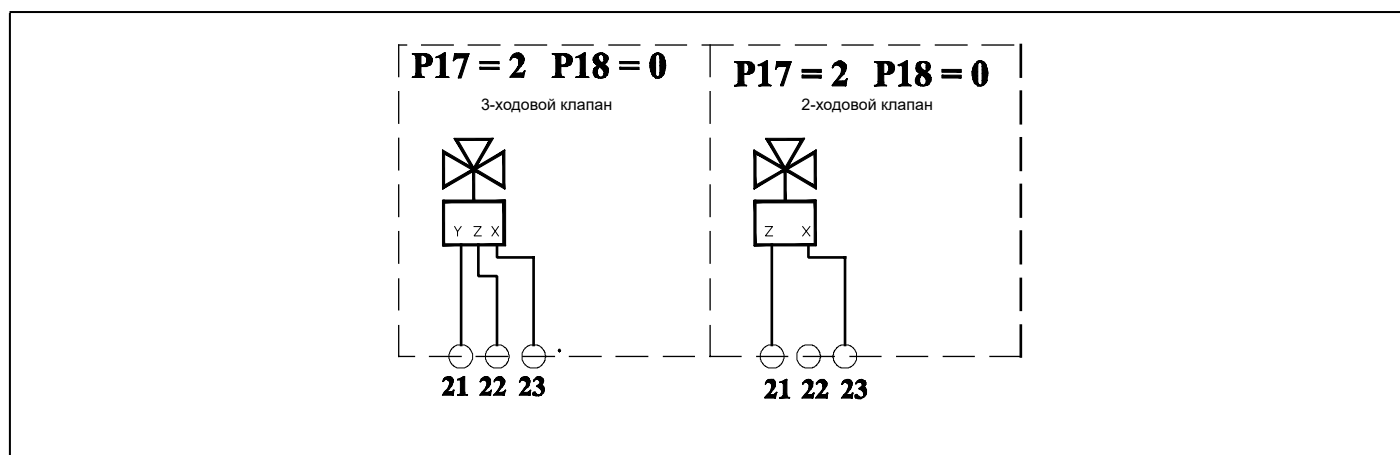
Рис. 28 Схема подключения многофункционального реле (X = общий; Y = на котел; Z = на коллектор)
