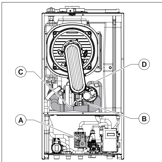
Рис. 36 Воздуховод
