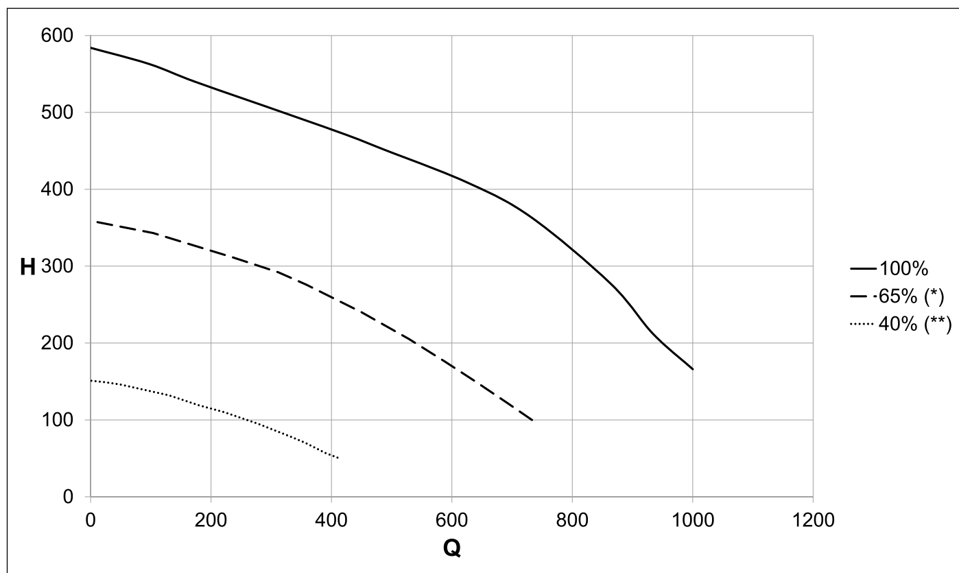
Рис. 20 Располагаемый напор KC-KR-KRB 12
