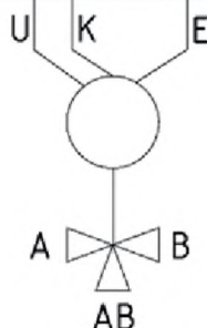
Рисунок 24 - Электроподключение привода трехходового клапана
