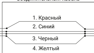
Соединительный кабель
