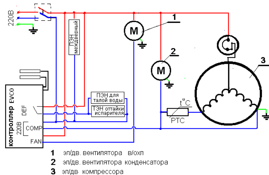
17.2 Электрическая схема стола ВТ.
