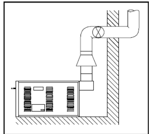
Рисунок 12 – Принудительный дымоотвод
