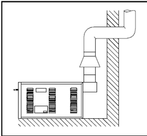
Рисунок 11 – Естественный дымоотвод
