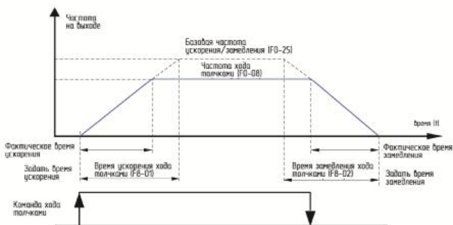
Рис. 5-13. Задание функции хода толчками
