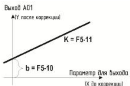
Рис. 5-32. Задание "k" и "b" выхода AO1
