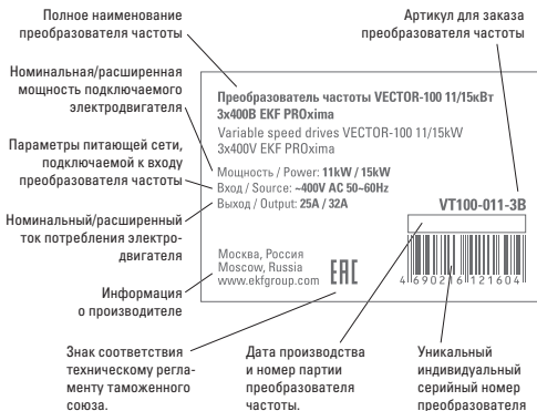
Рис. 2-2 Паспортная табличка.
