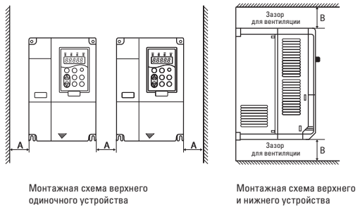
Рис. 4-1 Монтажная схема
