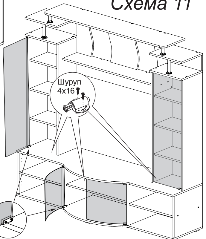
Схема установки стекловорки №26 и №27 в стеклопетлю
