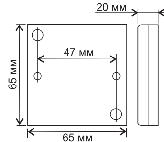
Рис.2 Габариты изделия.
