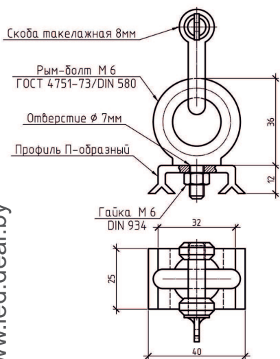
Крепление КПУ-25 (на трос)
