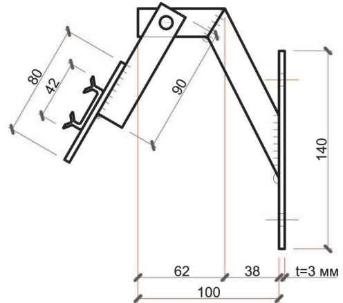
Крепление КПГ (поворотное)
