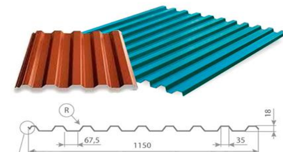
Кровельный профнастил МП-20
